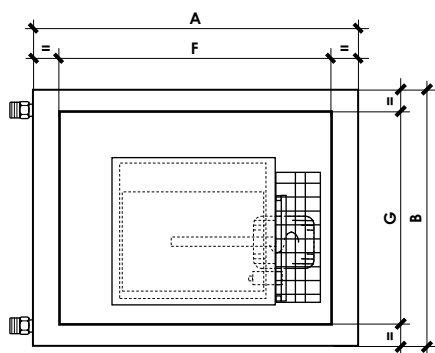
Bocca di aspirazione (attacco canale a baionetta) Air intake inlet (duct nesting connection)
